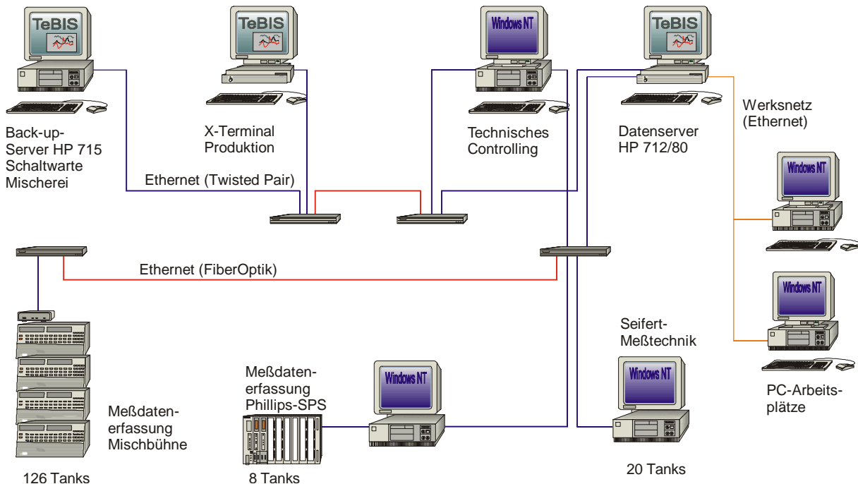
Hardware-Struktur des TeBIS â -Systems bei The Burmah Oil (Deutschland) GmbH
